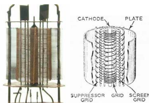
Fig.2. Aspecto interno del EL11. Colocación de las rejillas en un pentodo.
