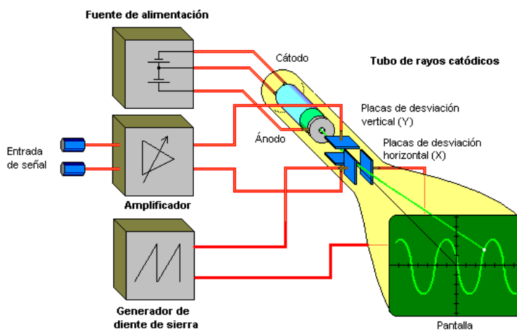
Figura 4. Representación esquemática de un osciloscopio.
